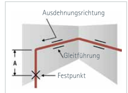
Bild 6.4 Anordnung von Rohrschellen bei Umführungen (3533)
