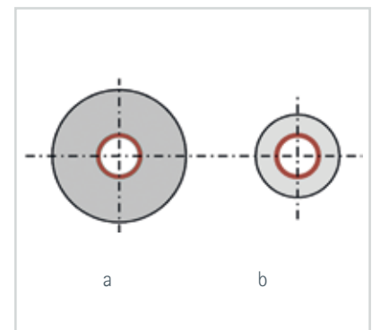
Bild 6.1 Vergleich des Platzbedarfs von werkseitig und bauseits wärmegeämmten Kupferrohren (6366)
