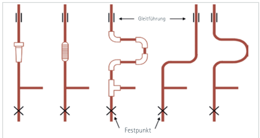
Bild 6.5 Ausdehnungsmöglichkeiten bei Rohrleitungen (4761)
