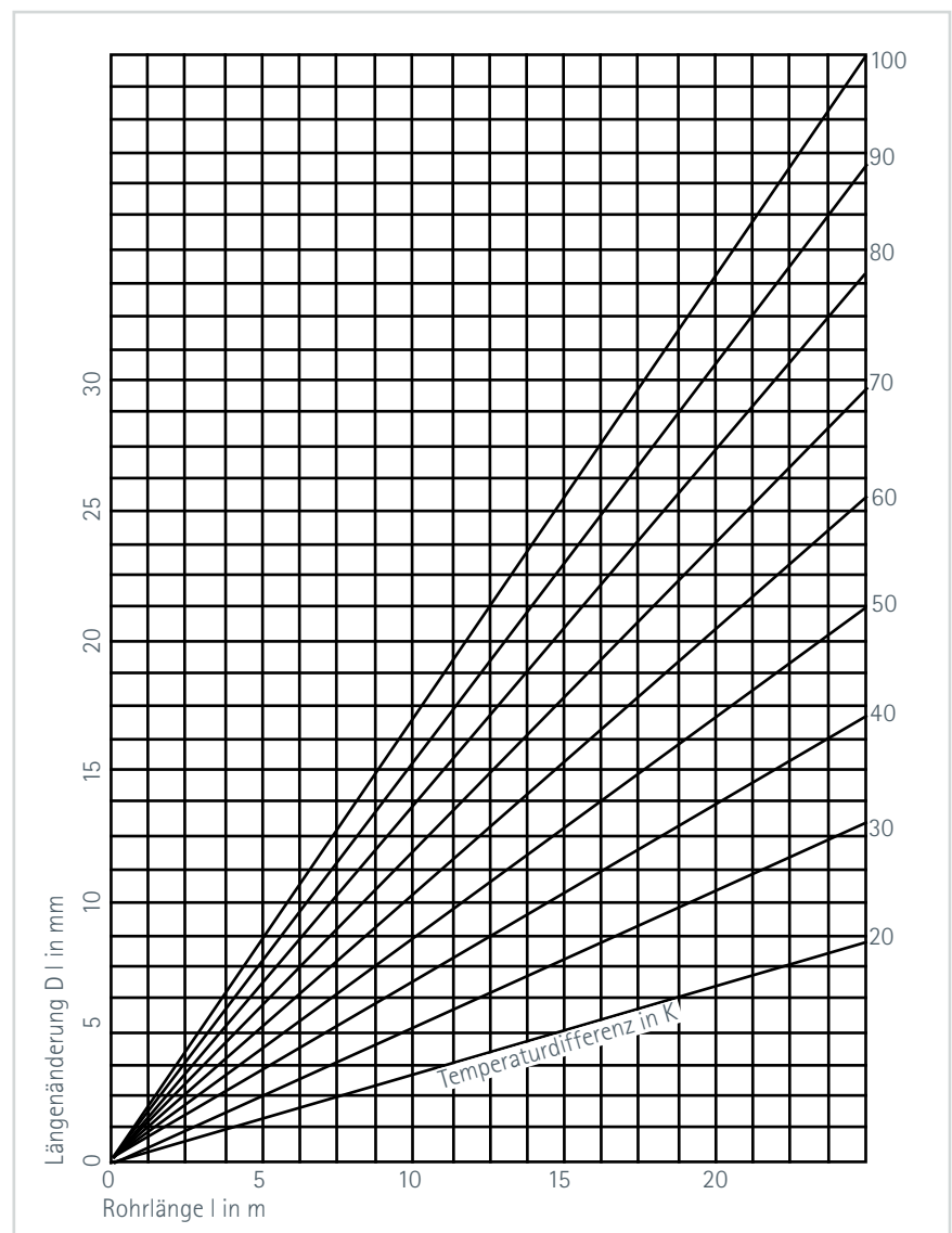
Bild 6.2 Temperaturbedingte Längenausdehnung von Kupferrohren in Abhängigkeit von der Rohrlänge (3679)
