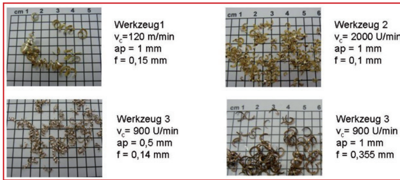
Bild 1: Späne von BlueBrass®42 nach Drehen mit verschiedenen Parametern
