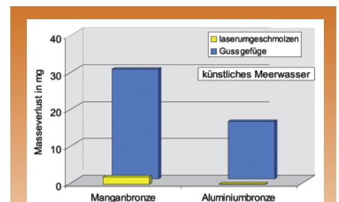
Bild 2: Verringerung des Masseverlustes infolge Kavitationserosion von Propellerbronzen nach Laserflächenbehandlung
