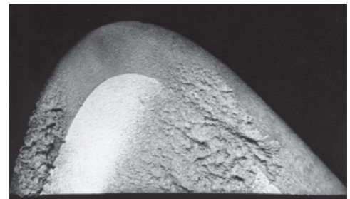
Bild 1: Durch Kavitationserosion geschädigte Spitze eines Schiffspropellers
