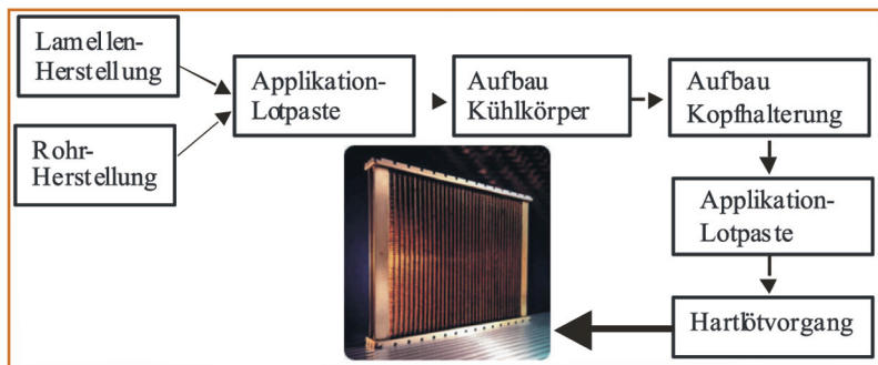
Bild 1: Cupro-Brazo® Verfahren
